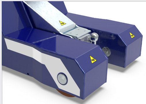
GANCIO CON ATTACCO A SFERA (BLOCCO FRONTALE)
