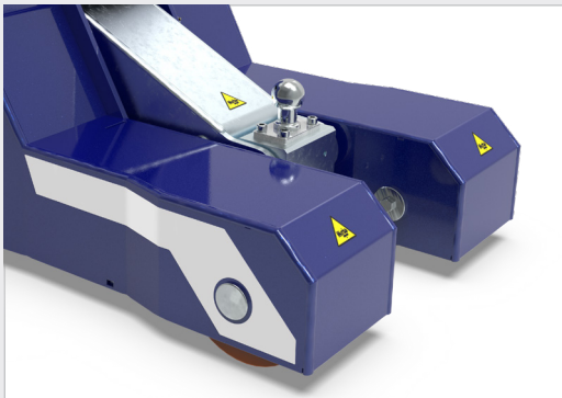
GANCIO A SFERA (BLOCCO SUPERIORE)
